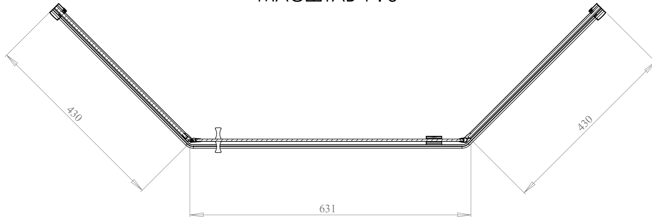
СЕЧЕНИЕ А-А МАСШТАБ 1 : 5
