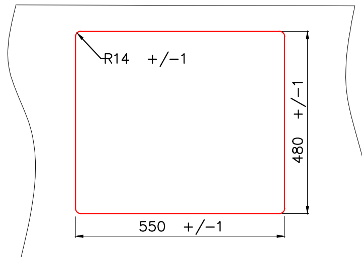
Врезной монтаж мойки (I)
