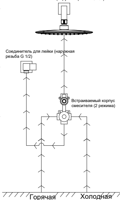
Схема установки водопроводной трубы
