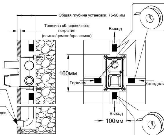
Встраиваемый корпус смесителя с блоком
