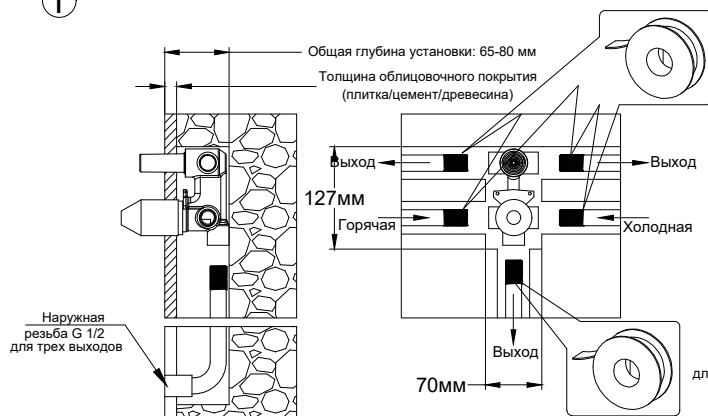
Встраиваемый корпус смесителя без блока
