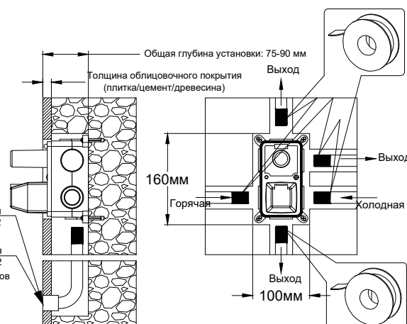
Встраиваемый корпус смесителя с блоком
